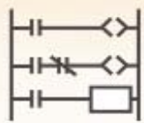
1 种编程语言
